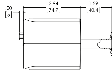
NW-KF-16
